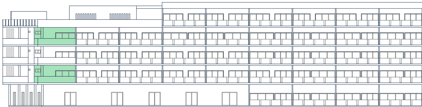
Fachada Norte
