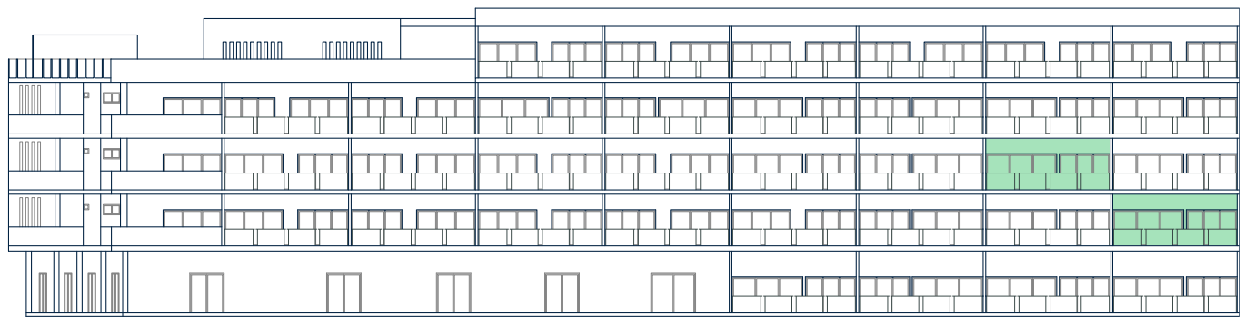
Fachada Norte
